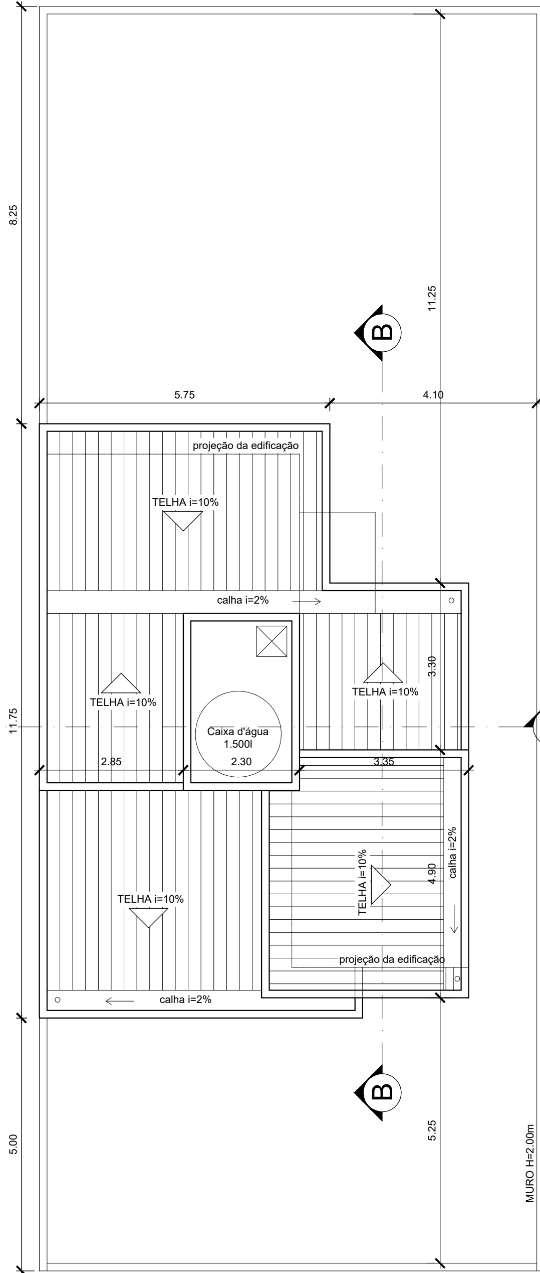
2 PLANTA DE COBERTURA ESCALA: 1/75
