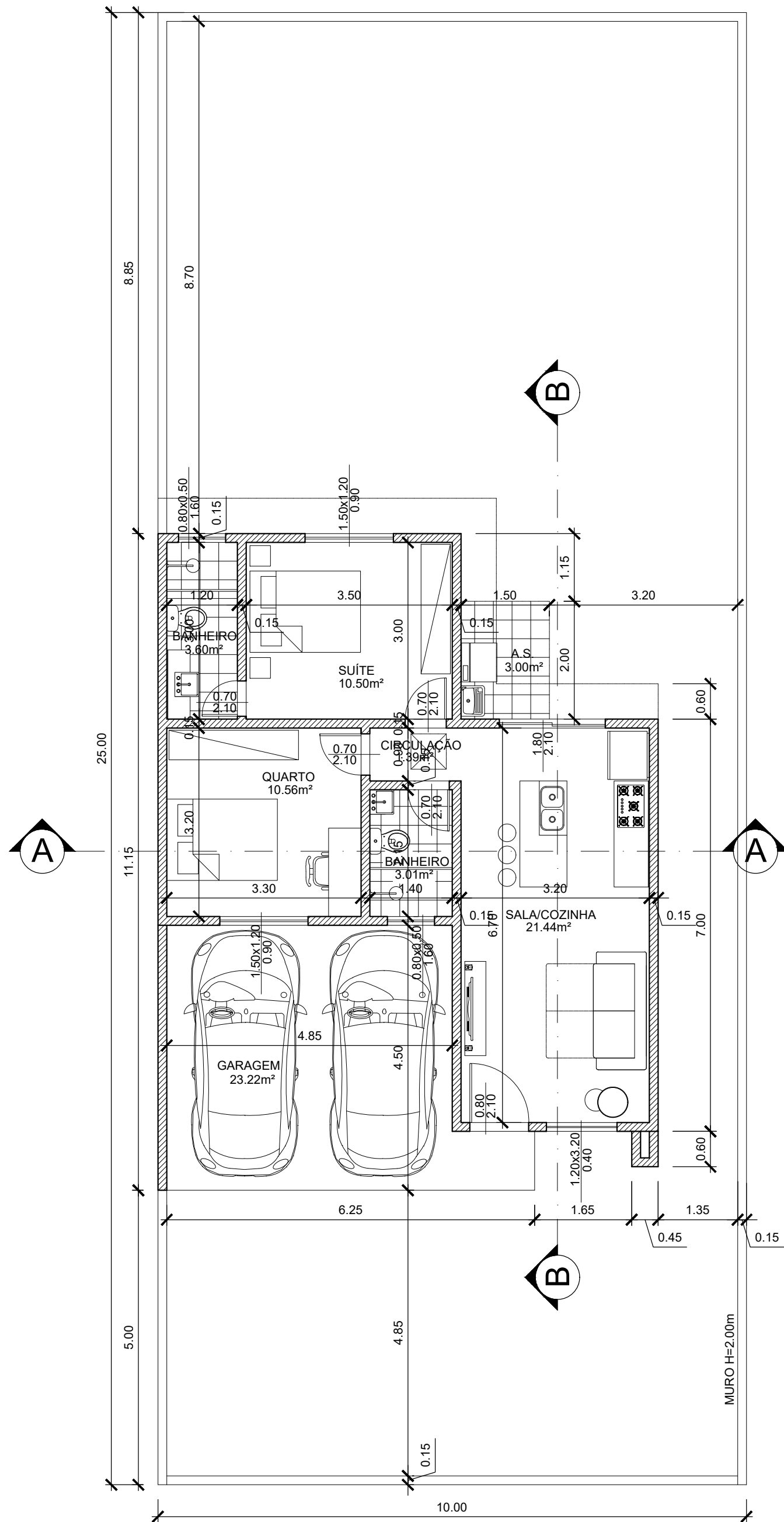
1 PLANTA BAIXA ESCALA: 1/75
