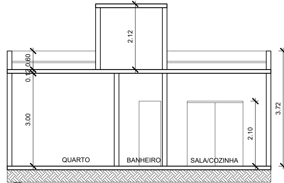
3 CORTE AA ESCALA: 1/75
