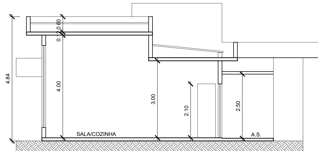
4 CORTE BB ESCALA: 1/75
